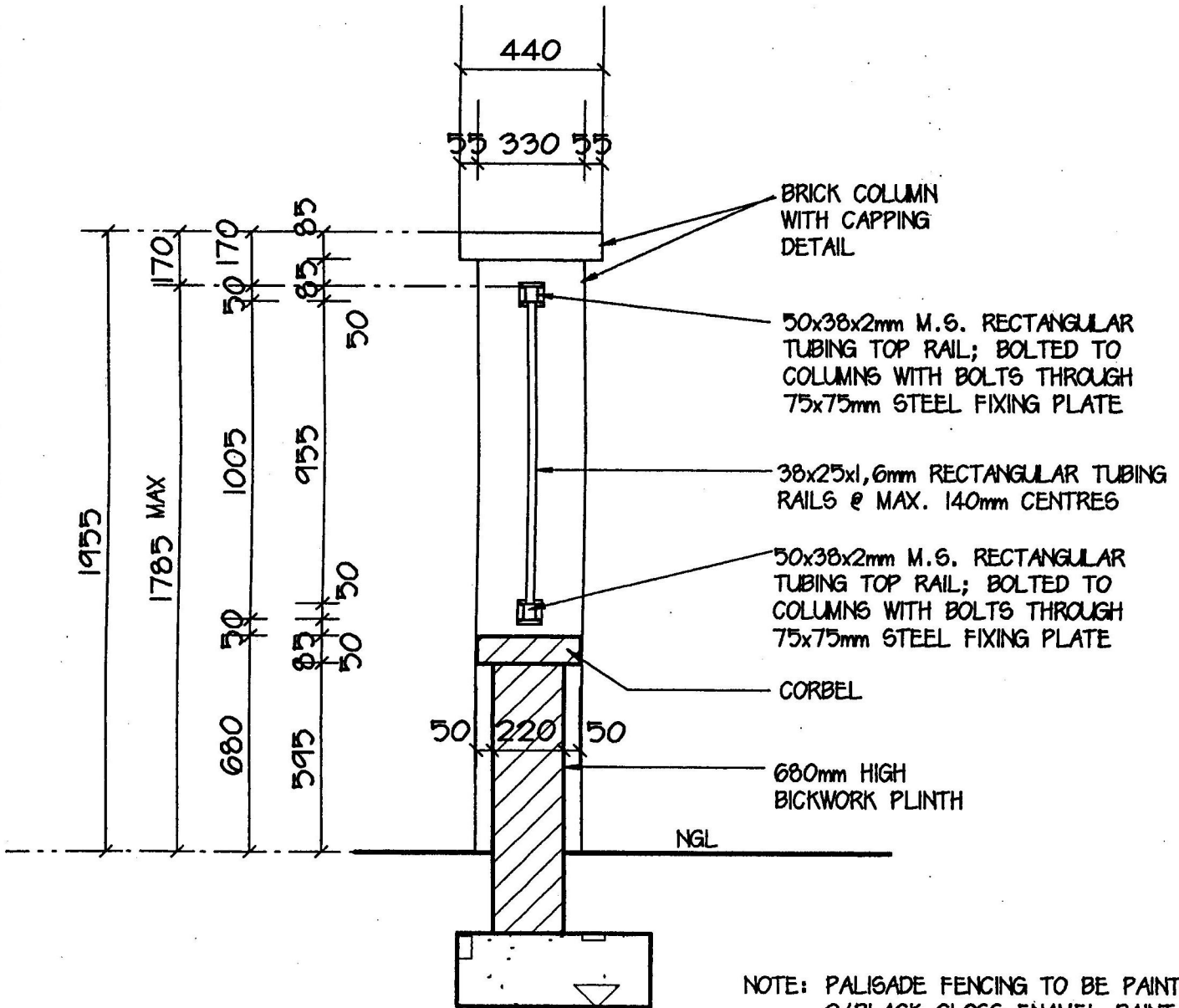
SECTION A-A
